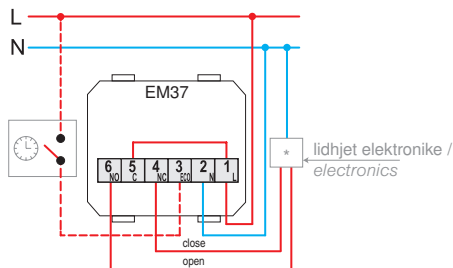
transmisioni me motor (përdorim i kufizuar me ngrohje nën dysheme) / motor drive (limited use with underfloor heating)
