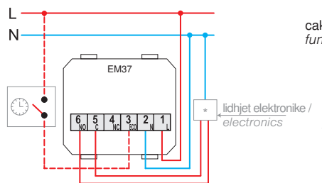
bojleri, pompa e nxehtësisë, vatra (hyrja e kontrollit T1/T2) / boiler, heat pump, burner (control input T1/T2)
